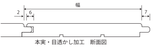
【共通断面図】
