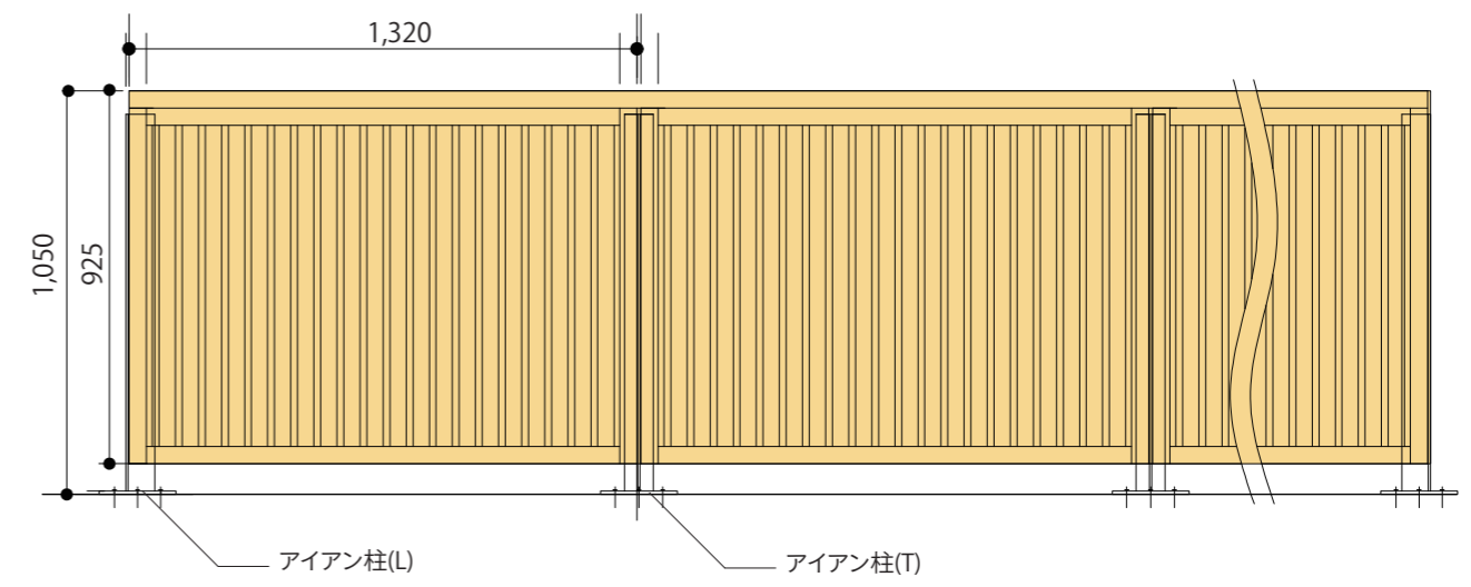
【木塀 参考図】 木塀パネル：W1320×H925
